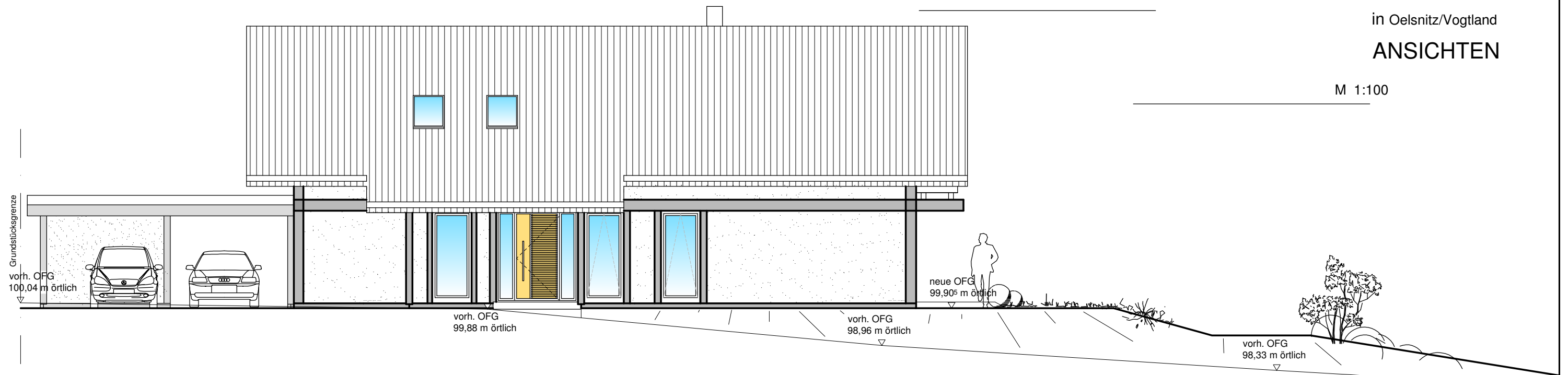
ANSICHT NORD-OST
