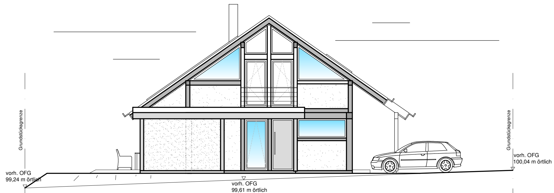
ANSICHT SÜD-OST
