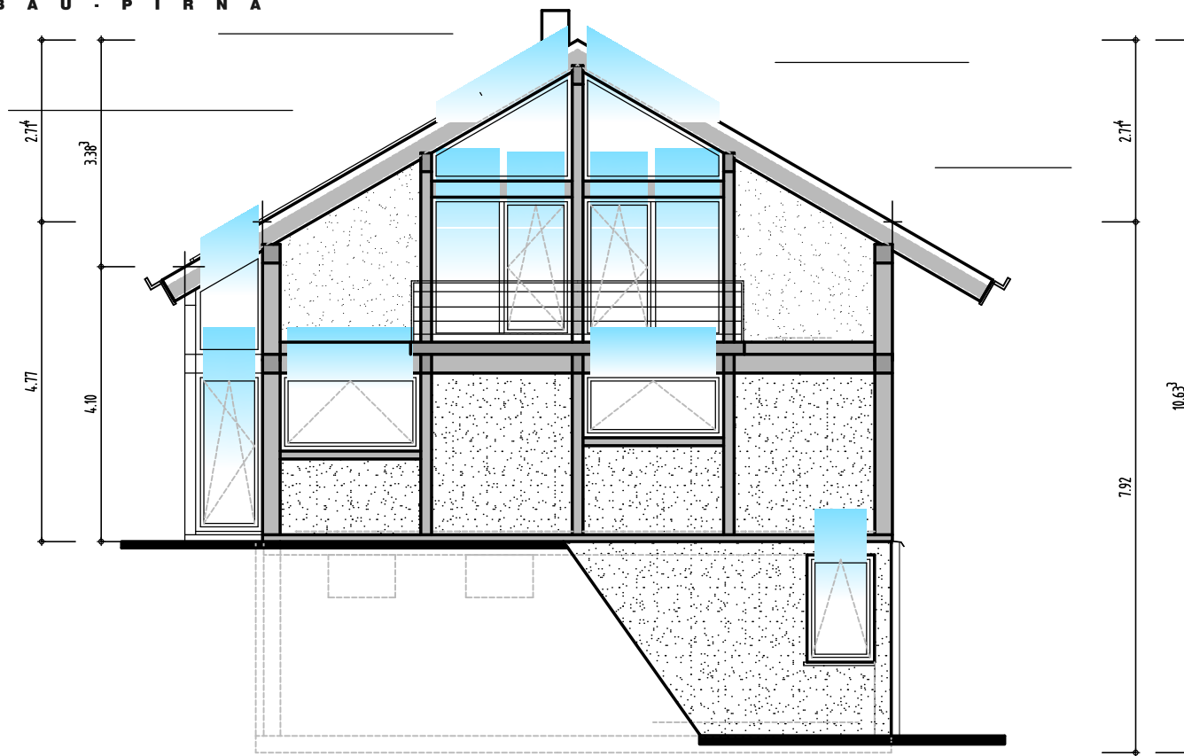
ANSICHT OST
