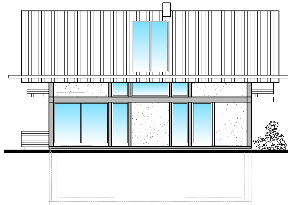
ANSICHT SÜD
