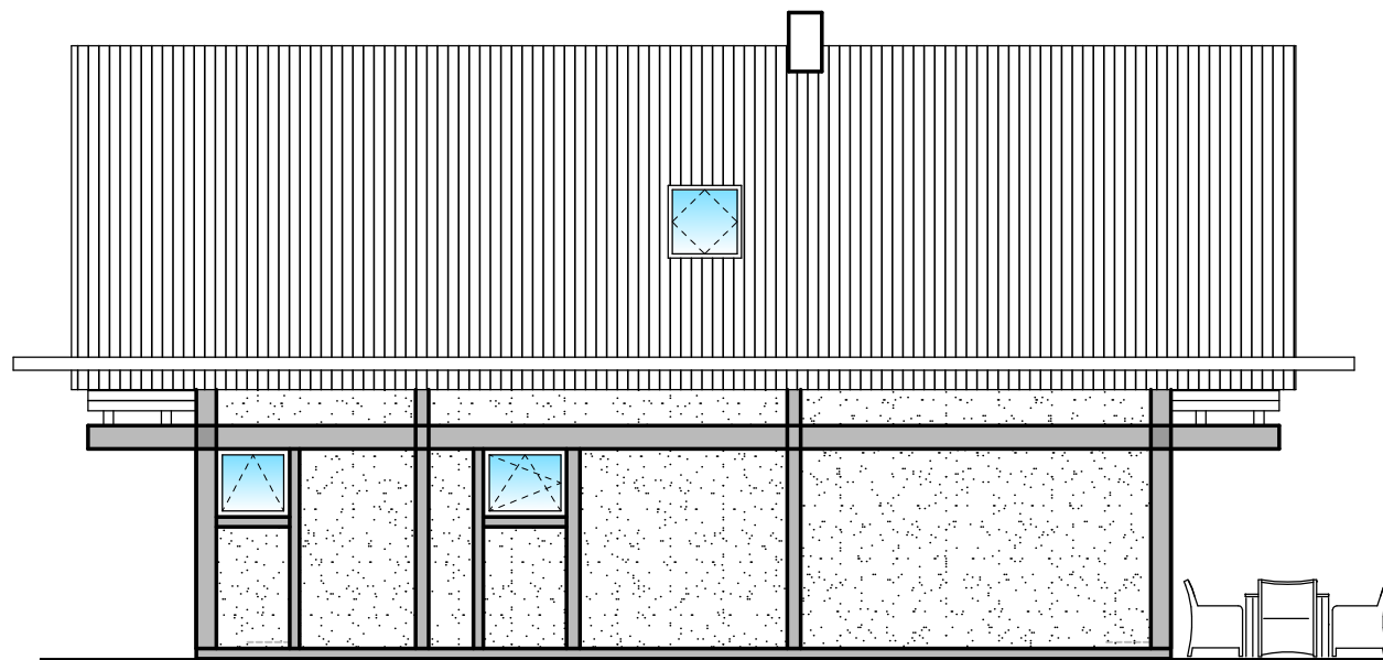
Ansicht Nord - West
