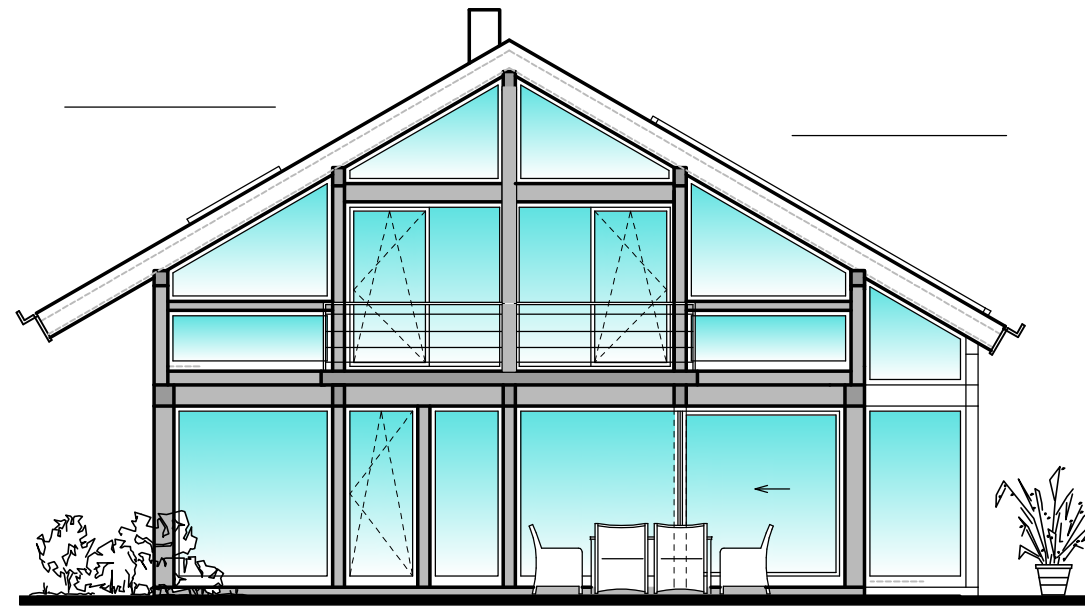
Ansicht Süd -West
