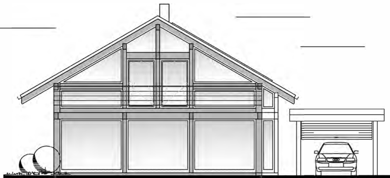
Ansicht West
